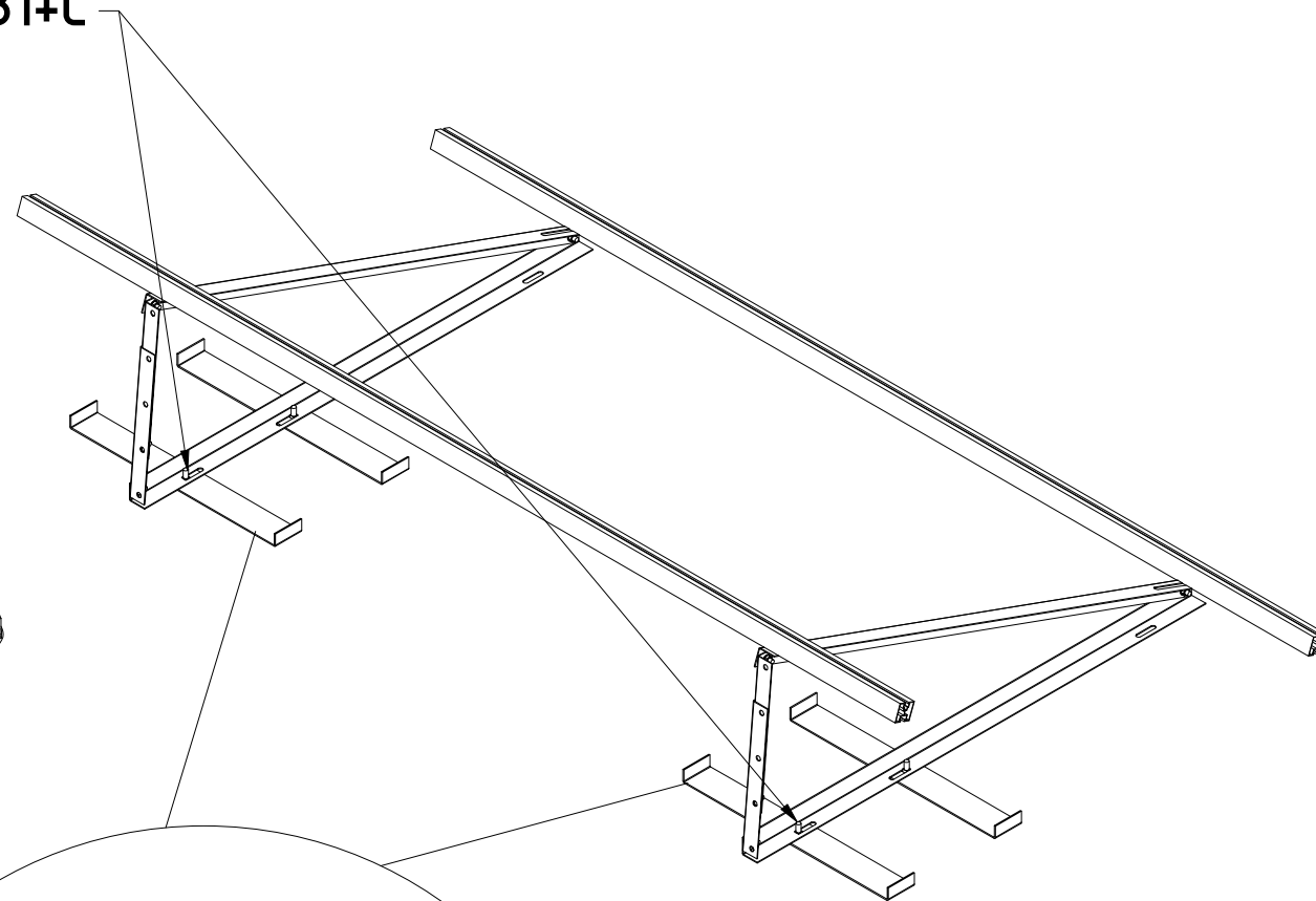
Rys.6 Wygląd konstrukcji wsporczej - wersja balastowa
