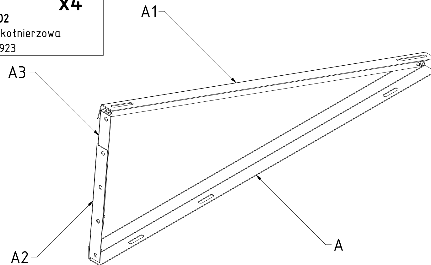
Rys. 1 Konstrukcja wsporcza - Złożenie
